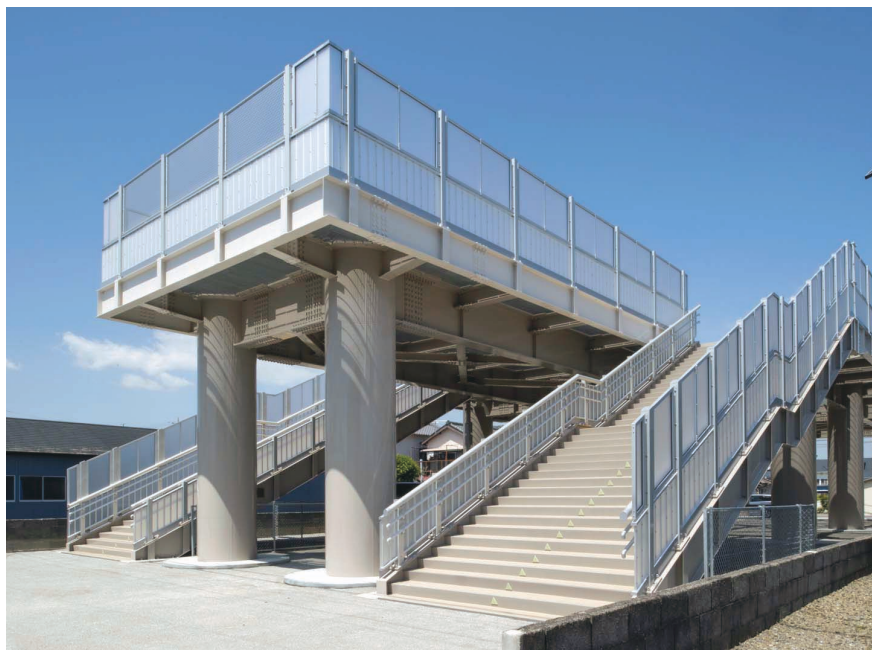
吉田町津波避難タワー（静岡県）／P工区
