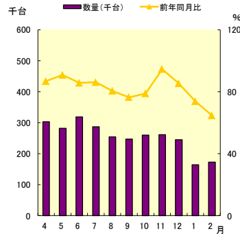
デジタルカメラ生産量
