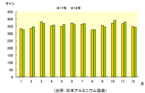
アルミニウム需要推移(月別)
