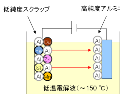
低温型電解法のイメージ図
